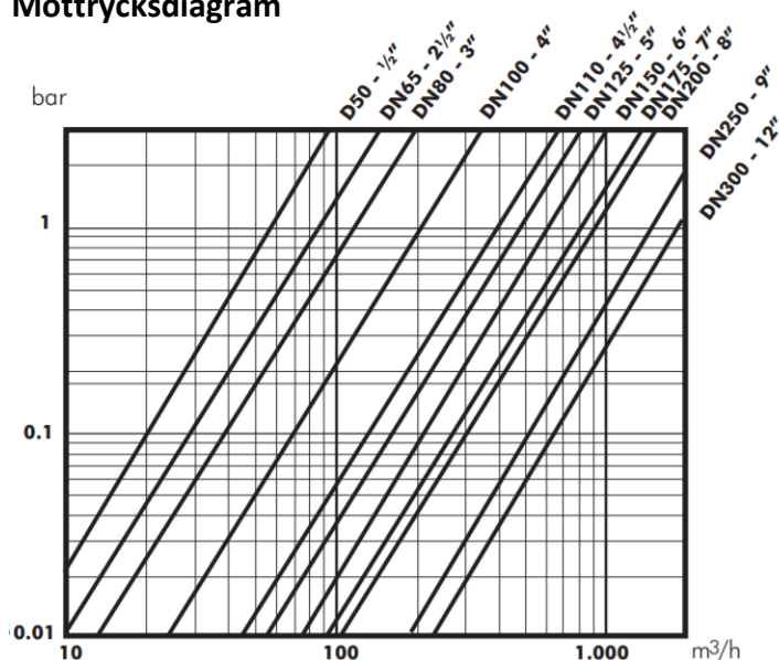
Mottrycksdiagram
